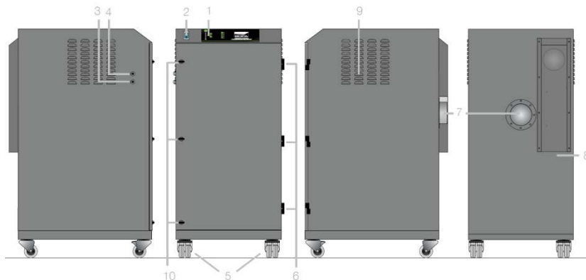
Внешний вид дымоуловителя AD 600-HP
